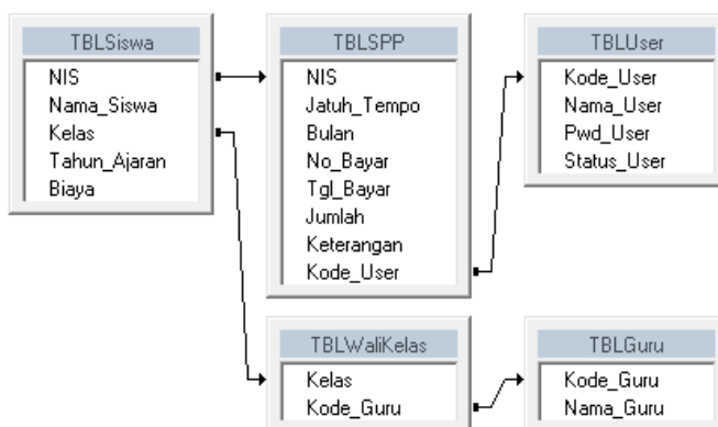
Relasi tabel aplikasi pembayaran SPP
